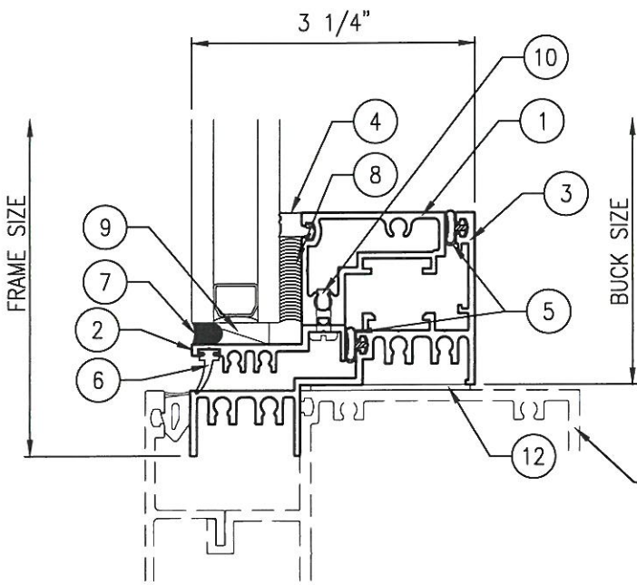
2 SILL - FRAME ASSEMBLY Scale: 6" = 1'-0"
