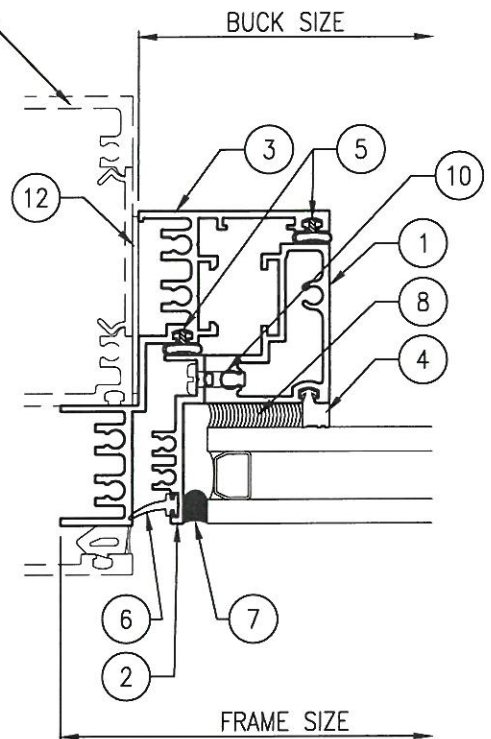
3 JAMB - FRAME ASSEMBLY Scale: 6" = 1'-0"
