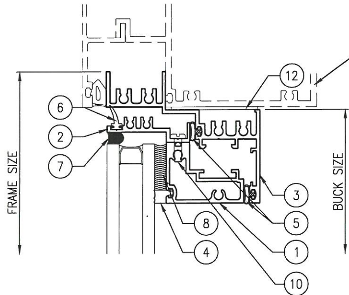
1 HEAD - FRAME ASSEMBLY Scale: 6" = 1'-0"
